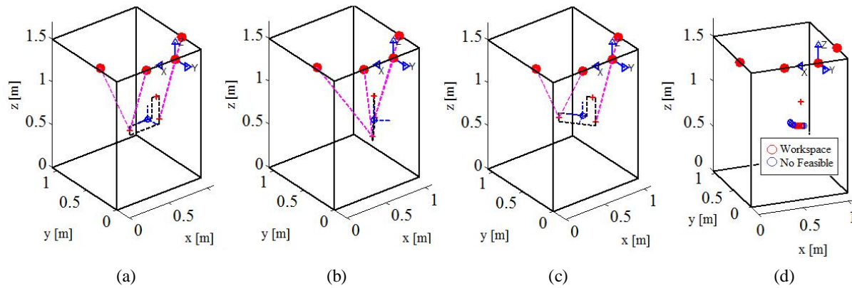
Figure 11. (a) Splint the initial position 0^\circ ; (b) Rotation in z 50^\circ ; (c) Rotation in z -50^\circ ; (d) Workspace.
