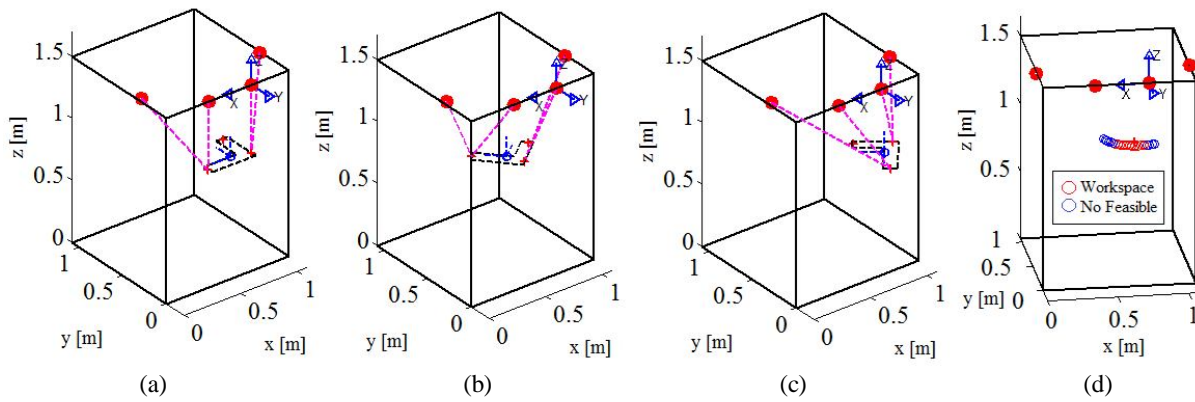
Figure 10. (a) Splint the initial position 90^\circ ; (b) Horizontal flexion -50^\circ ; (c) Horizontal extension 50^\circ ; (d) Workspace.
