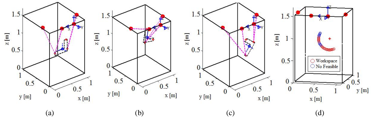
Figure 9. (a) Splint the initial position 0^\circ ; (b) Vertical flexion -100^\circ ; (c) Vertical extension 50^\circ ; (d) Workspace.
