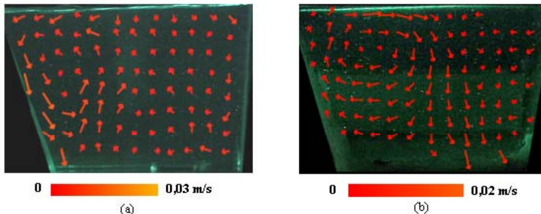
Figura 4.1. Campos de velocidade para PL1: (a) sem modificadores de escoamento, (b) com modificadores de escoamento.
