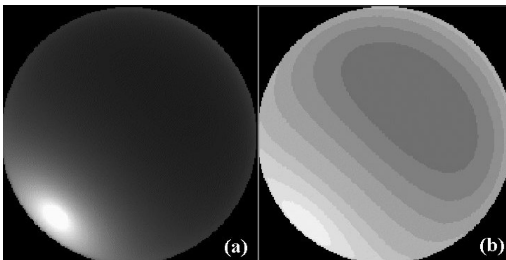
Figura 4. Simulação de resultados para o modelo CIE: (a) céu limpo; (b) seu respectivo mapa de tons de cinza.
