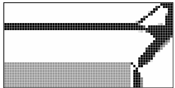
(f) w = 0,8 ; V^* = 15\% ; 2500 elements
