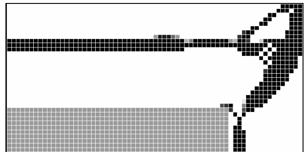
(d) w = 0,8 ; V^* = 15\% ; 2500 elements and filter turn off
