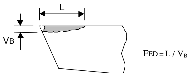
Figura 2 - Relação entre o desgaste ao longo da aresta ( L ) e da superfície de folga ( V_B ).
