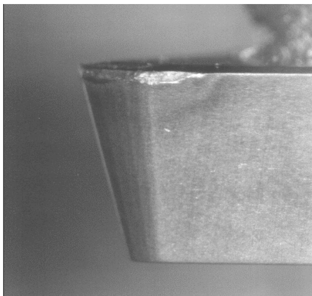
Figura 3 - Pastilha não lapidada após o último período de ensaio (aumento de 25 vezes).
