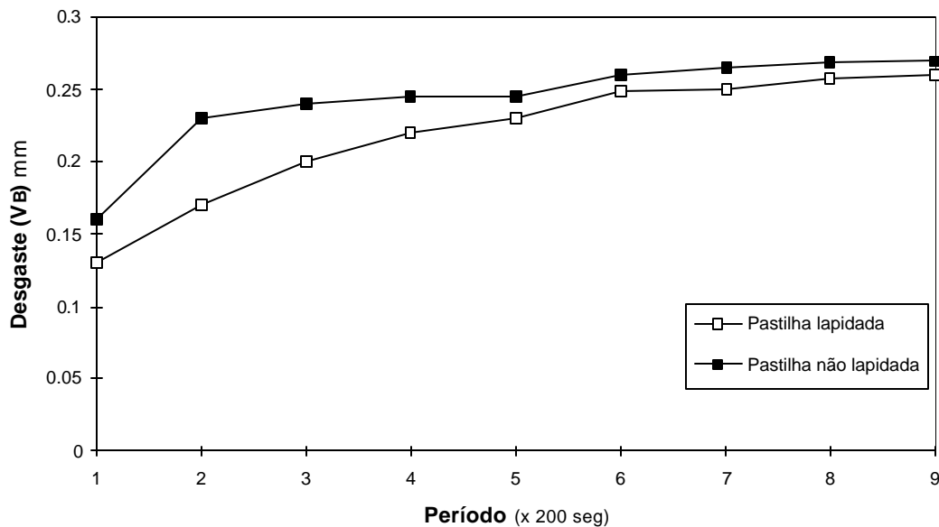
Figura 5 - Desgaste da superfície de folga ( V_B ) em pastilhas de metal duro lapidadas e não lapidadas ao final de cada período.
