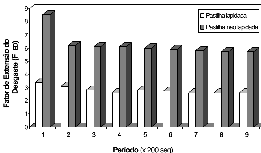
Figura 6 - “Fator de Extensão do Desgaste ( F_{ED} )” para as pastilhas de metal duro lapidadas e não lapidadas.
